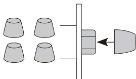
Fissaggio dei cappucci del mozzo
